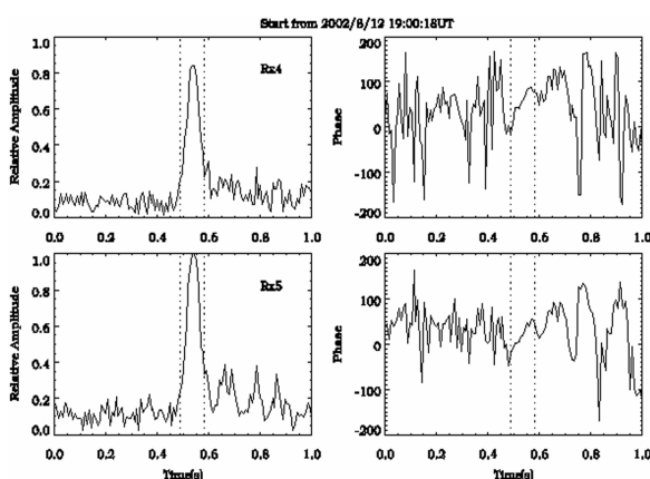
图1 2002年8月13日两个接受通道上一个流星回波的振幅和相位
